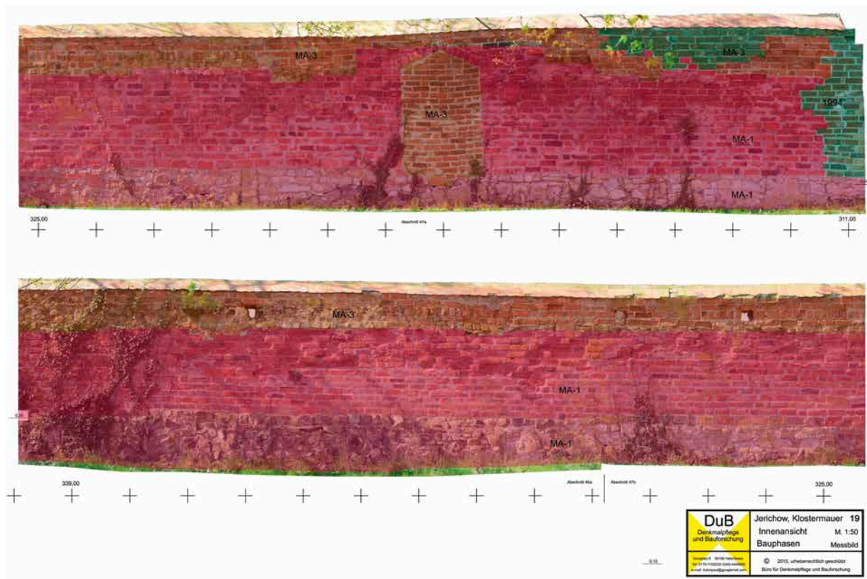
ABB. 2 Südwestliche Klostermauer mit ältestem Backsteinmauerwerk, Innenseite, Abschnitt 47i–48i (MA-1) und bauzeitlicher Tür, vermauert bereits mit dem spätromanischen Mauerwerk MA-3 (Dokumentation von Maurizio Paul, 2015)
